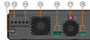
(2KW-3KW model)
